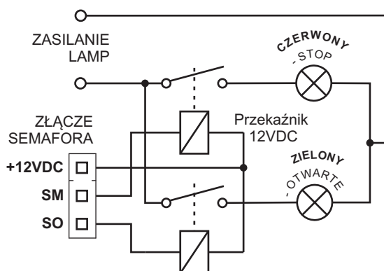
Rysunek 4. Sposób podłączenia dodatkowej sygnalizacji świetlnej
