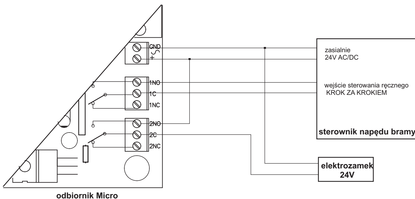
Rys.2 Przykładowy schemat elektryczny połączenia odbiornika MICRO z centralą sterownika bramowego oraz elektrozamkiem.
