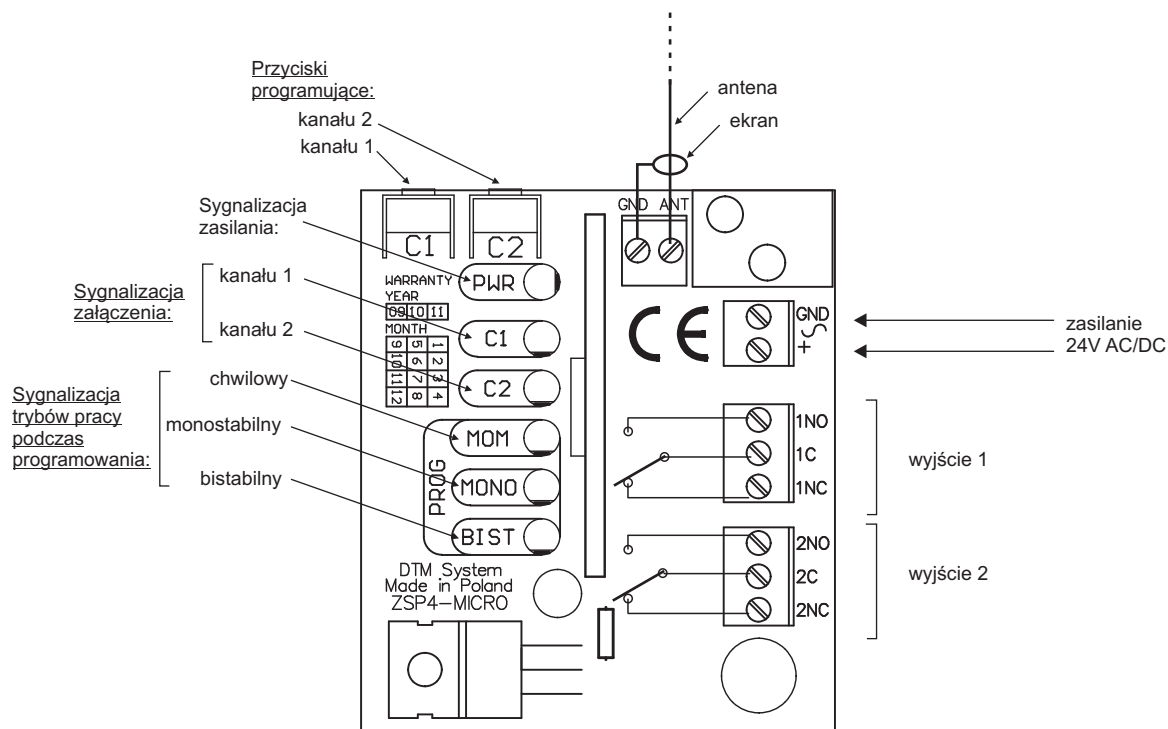
Rys. 1 Schemat płyty odbiornika
